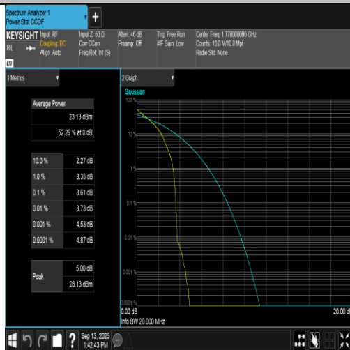
Band66-20MHz-QPSK-132572-1RB#0-PASS
