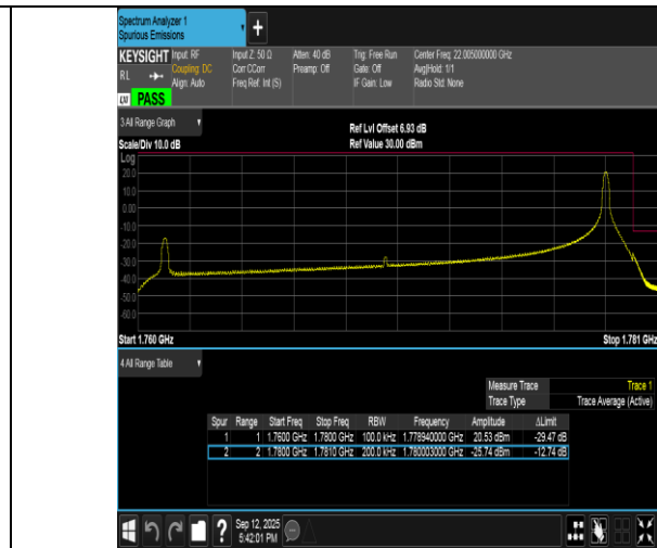
Band66-20MHz-QPSK-132572-1RB#99-PASS
