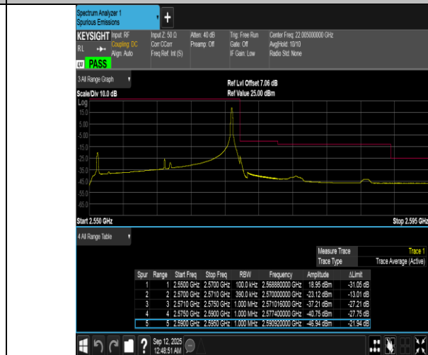
Band7-20MHz-QPSK-21350-1RB#99-PASS
