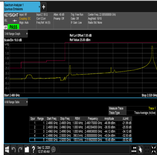
Band7-20MHz-QPSK-20850-1RB#99-PASS
