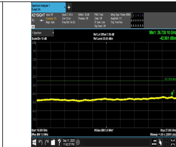
Band7-15MHz-QPSK-20825-1RB#0-18000~27000-PASS
