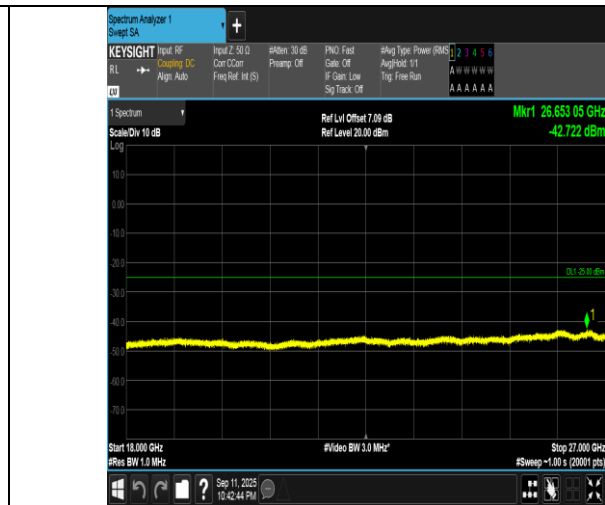
Band7-10MHz-QPSK-21100-50RB#0-18000~27000-PASS
