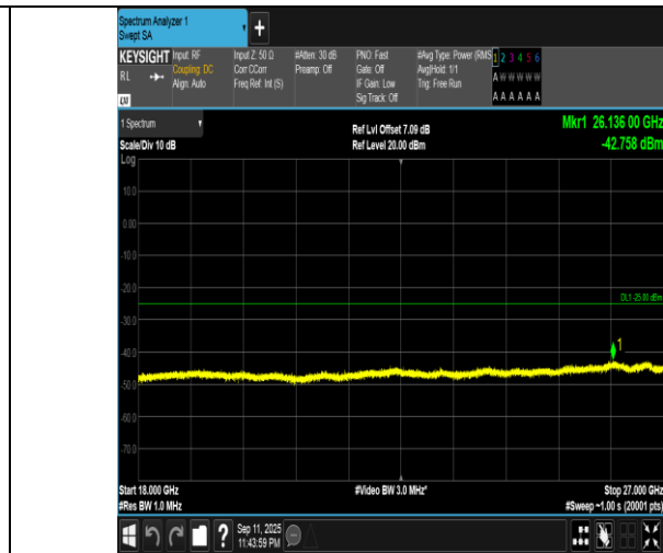
Band7-15MHz-16QAM-20825-1RB#0-18000~27000-PASS
