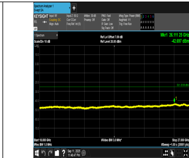
Band7-15MHz-16QAM-20825-1RB#74-18000~27000-PASS
