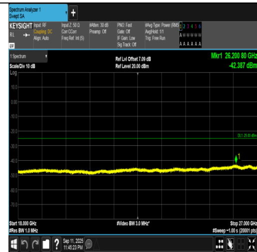
Band7-15MHz-QPSK-20825-1RB#74-18000~27000-PASS
