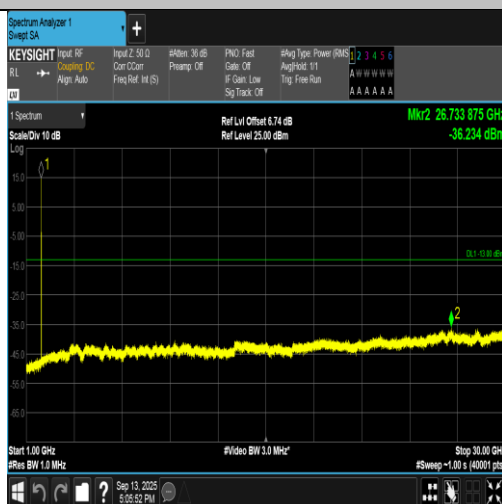
Band2-9538-4-1000~30000MHz-PASS
