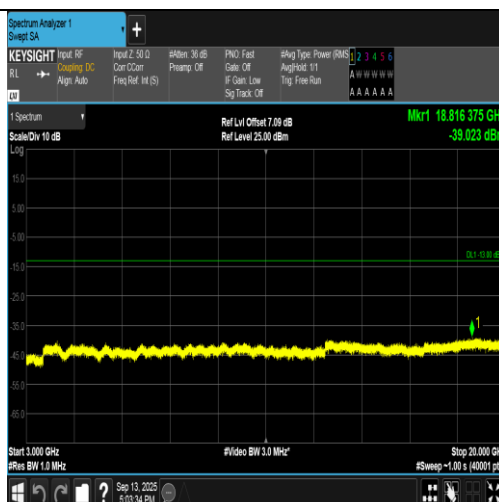
Band2-9538-3-3000~20000MHz-PASS
