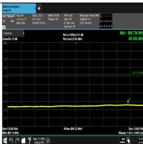
Band2-9538-1-30~1000MHz-PASS
