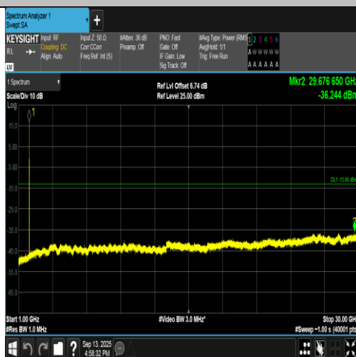
Band2-9538-1-1000~30000MHz-PASS
