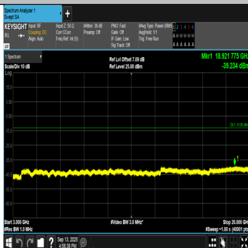
Band2-9538-1-3000~20000MHz-PASS
