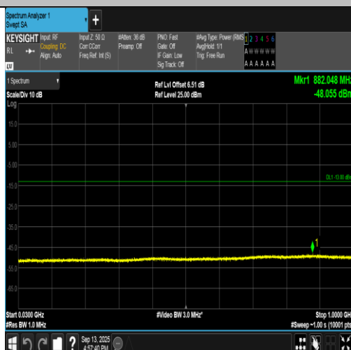
Band2-9400-1-30~1000MHz-PASS
