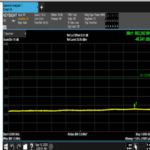
Band2-9538-2-30~1000MHz-PASS
