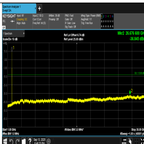
Band2-9538-3-1000~30000MHz-PASS
