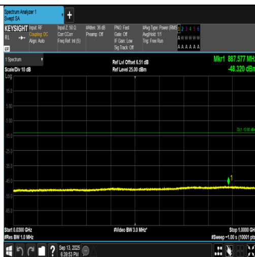
Band2-9400-1-30~1000MHz-PASS
