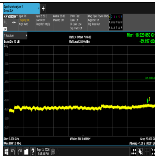
Band2-9400-3-3000~20000MHz-PASS
