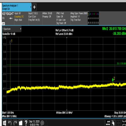
Band2-9400-1-1000~30000MHz-PASS
