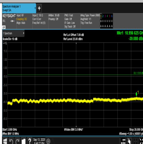
Band2-9538-3-3000~20000MHz-PASS
