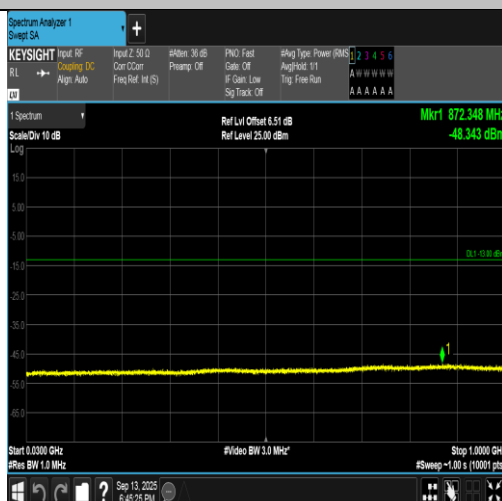
Band2-9400-3-30~1000MHz-PASS
