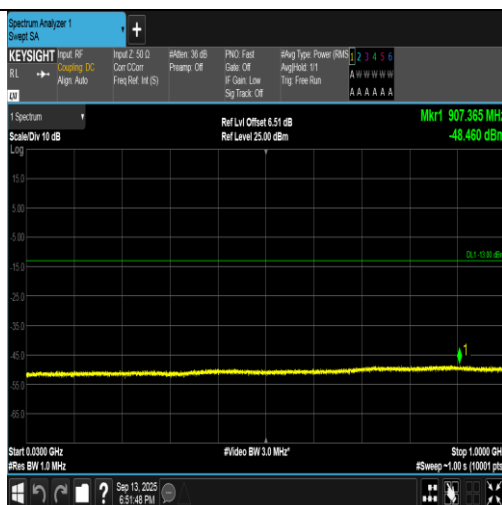
Band2-9538-5-30~1000MHz-PASS
