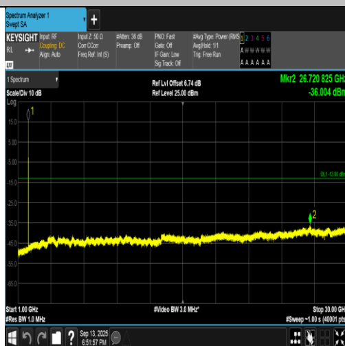
Band2-9538-5-1000~30000MHz-PASS
