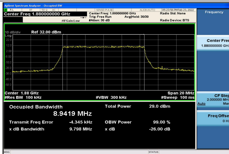
Band2-10MHz-QPSK-18900-50RB#0-8.9419
