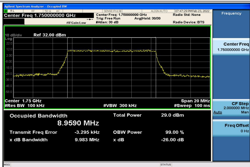
Band4-10MHz-QPSK-20350-50RB#0-8.9590
