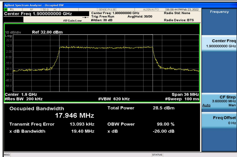
Band2-20MHz-16QAM-19100-100RB#0-17.946
