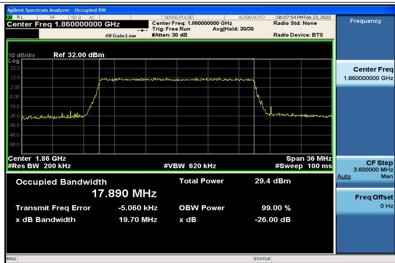
Band2-20MHz-QPSK-18700-100RB#0-17.890
