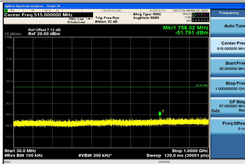
Band41-5MHz-QPSK-40065-1RB#0-30~1000MHz
