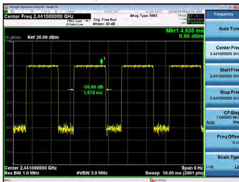
\pi/4 -DQPSK 2DH3 2441MHZ
