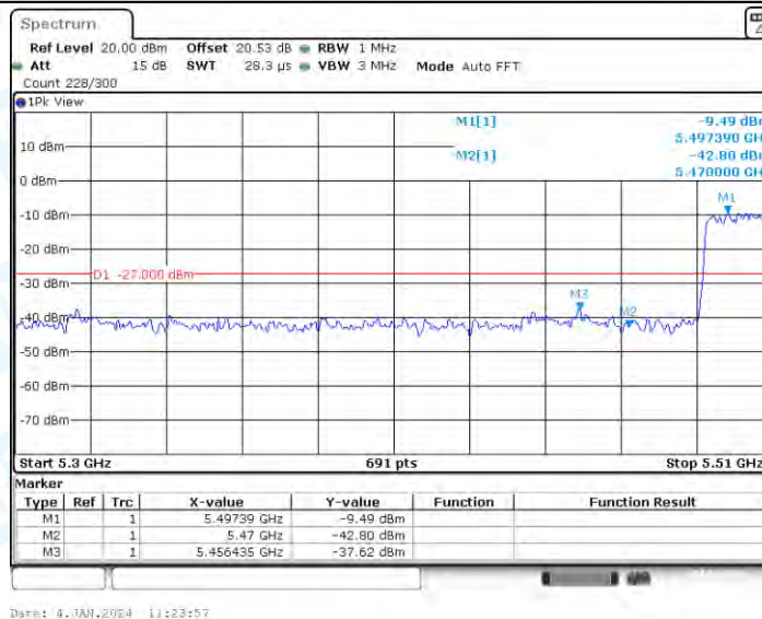
11N20MIMO_Ant2_Low_5500
