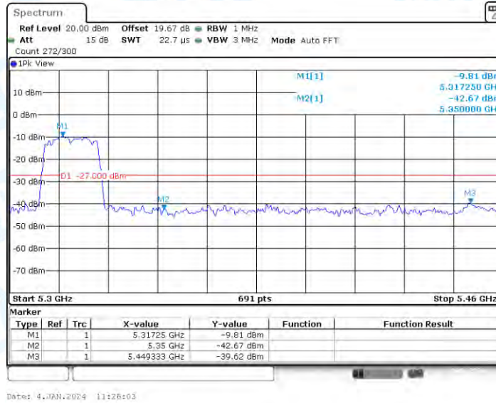
11N20MIMO_Ant2_High_5320
