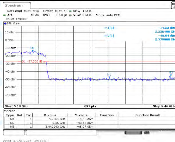
11AC80MIMO_Ant1_Low_5290
