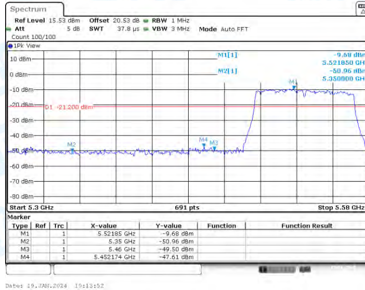
11AC80-MIMO_Ant2_Low_5530_AV
