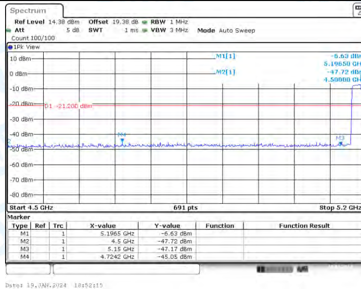
11AC40-MIMO_Ant2_Low_5190_AV
