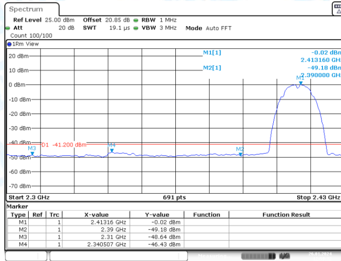
11B-CDD_Ant1_Low_2412_AV
