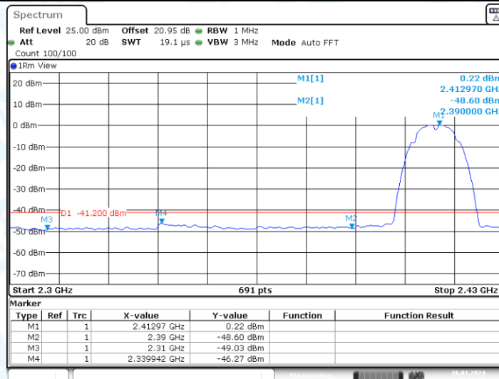
11B-CDD_Ant2_Low_2412_AV
