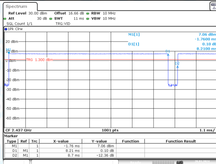
11B-CDD_Ant1_2437
