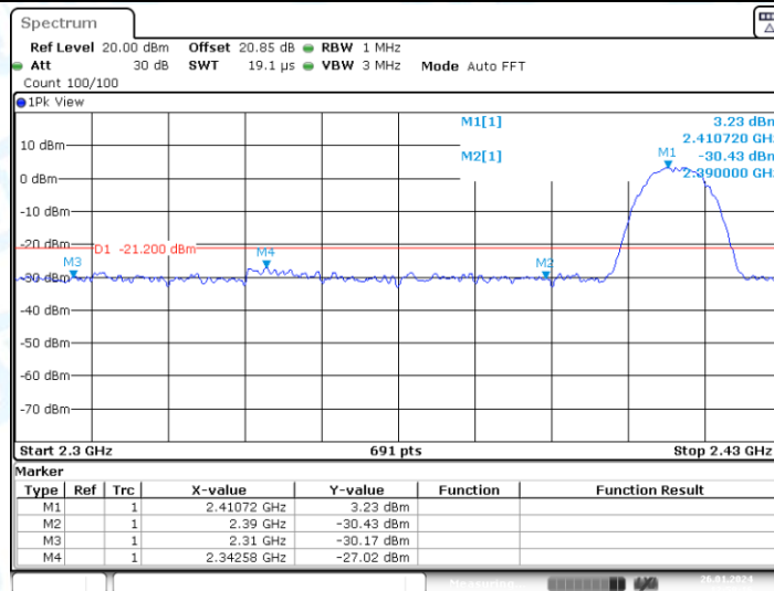
11B-CDD_Ant1_Low_2412_Peak
