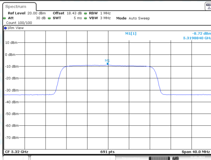
11AC20MIMO_Ant1_5320
