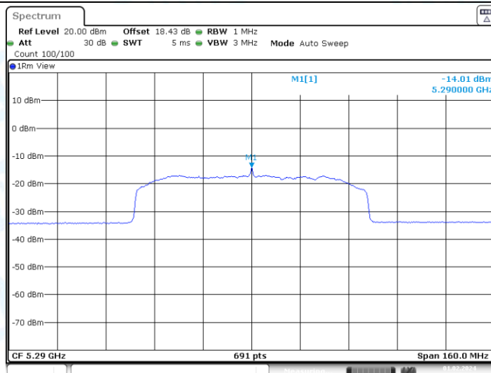
11AC80MIMO_Ant2_5290
