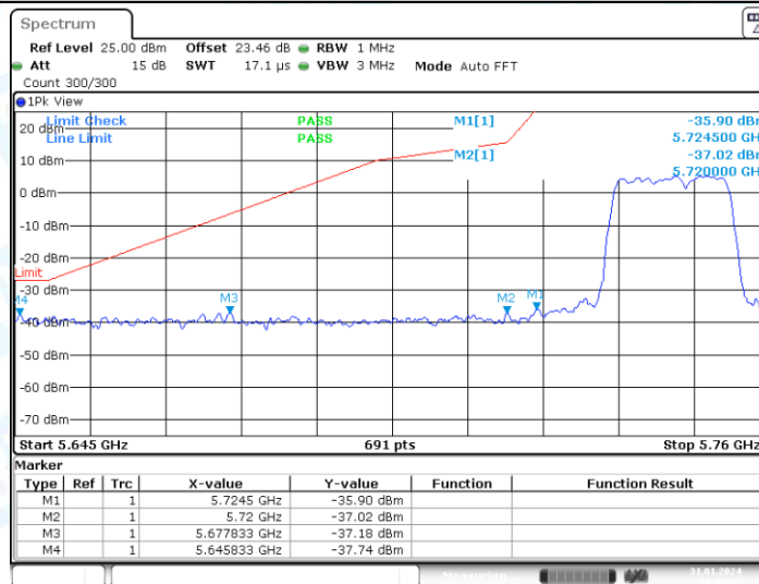
11N20MIMO_Ant2_Low_5745
