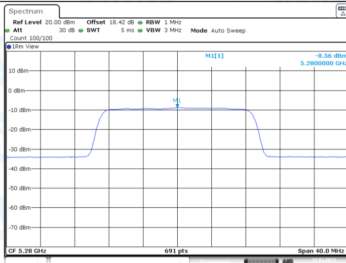
11AC20MIMO_Ant2_5280
