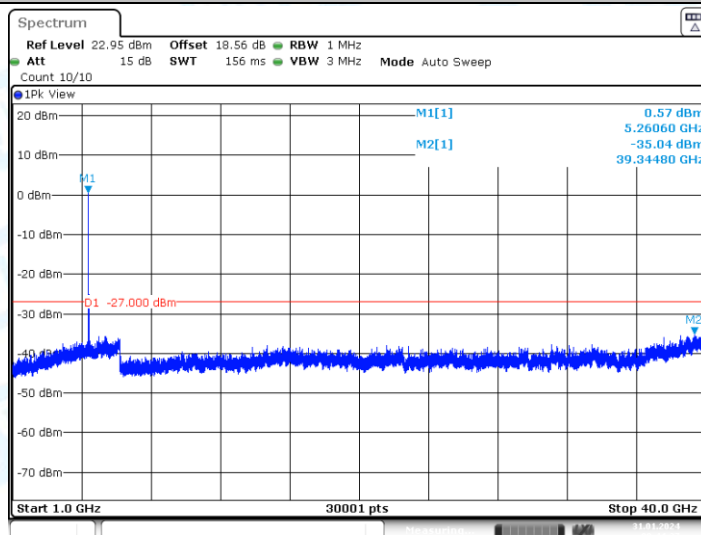
11N20MIMO_Ant2_5260_1000~40000
