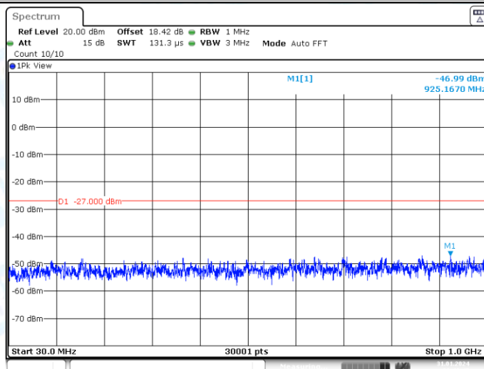
11N20MIMO_Ant1_5280_30~1000
