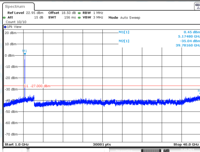
11AC20MIMO_Ant2_5180_1000~40000
