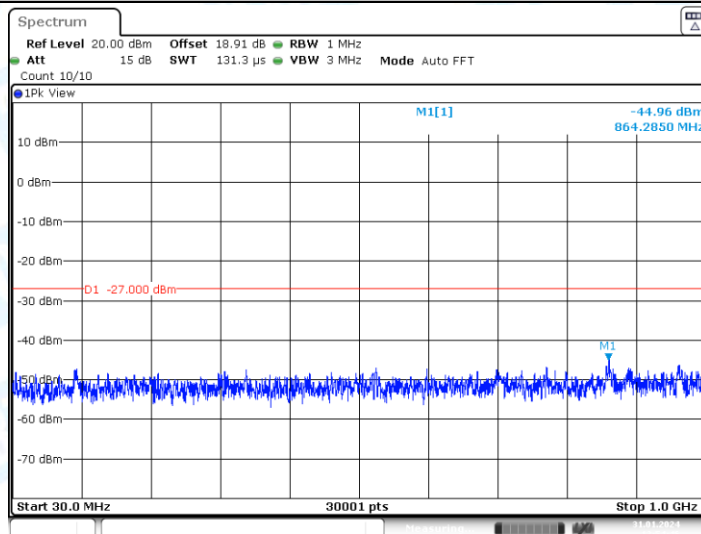
11AC20MIMO_Ant2_5700_30~1000
