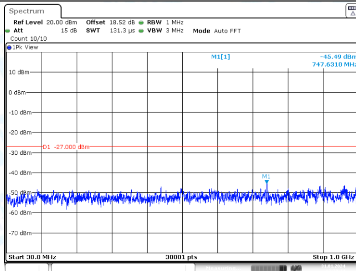
11AC20MIMO_Ant2_5320_30~1000
