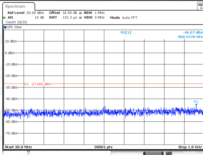
11AC20MIMO_Ant1_5580_30~1000
