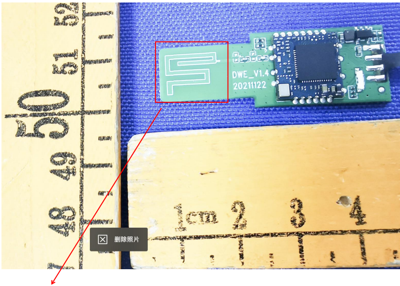
Antenna
