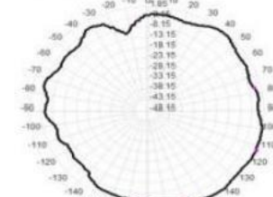
2402.0MHz Tota(E1),Max=1.85dB
