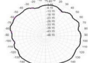
2402.0MHz Tota(E2),Max=-0.09dB
