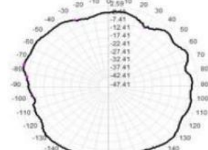
2441.0MHz Tota(E2),Max=-0.09dB
