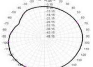
2402.0MHz Tota(H) Max=-0.06dB
