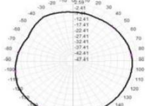
2441.0MHz Tota(F) Max=-0.06dB
