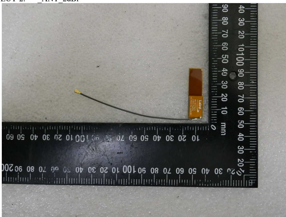
EUT-2. _ANT_2dBi
