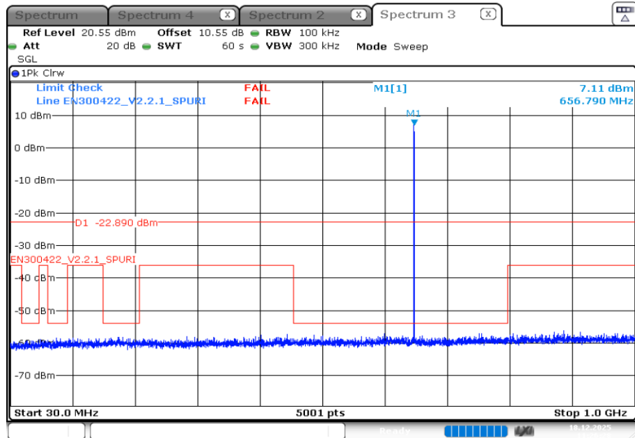
Plot 3: 656.8MHz, 30 MHz – 1 GHz
