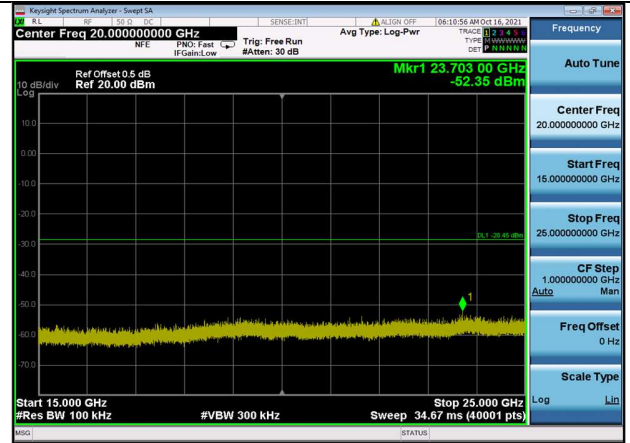
802.11n(HT20),2462MHz,Ant0,Plot 6,15000MHz~25000MHz
