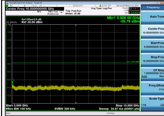
802.11n(HT20),2462MHz,Ant0,Plot 5,5000MHz~15000MHz
