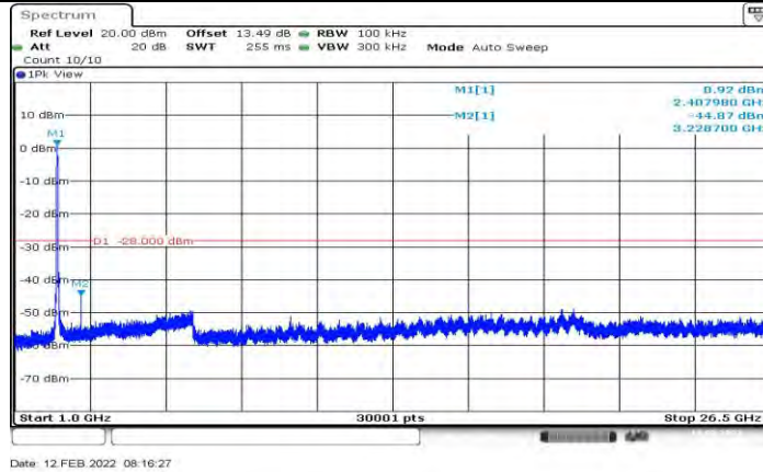
11N40SISO Ant1 2422_1000~26500
