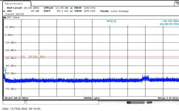
11N40SISO Ant1 2422_30~1000
