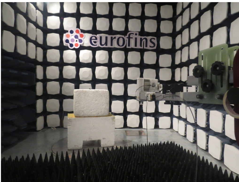
18GHz - 26.5GHz
