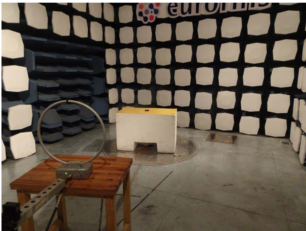
9kHz-30MHz
