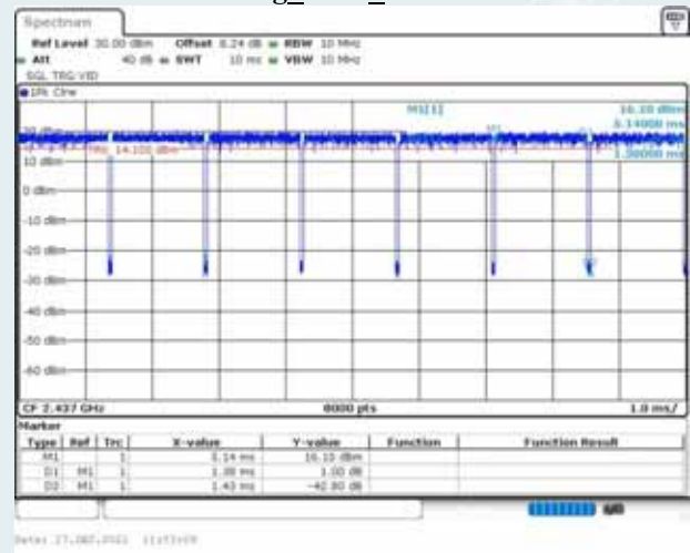
802.11g_Ant1_2437MHz
