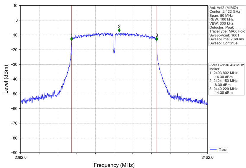
802.11n(HT40)_LCH_2422MHz_Ant2 (MIMO)_NTNV
