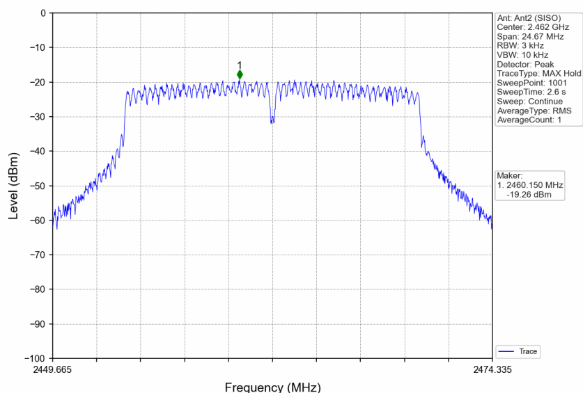
802.11g_HCH_2462MHz_Ant2 (SISO)_NTNV
