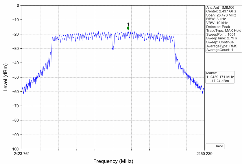
802.11n(HT20)_MCH_2437MHz_Ant1(MIMO)_NTNV
