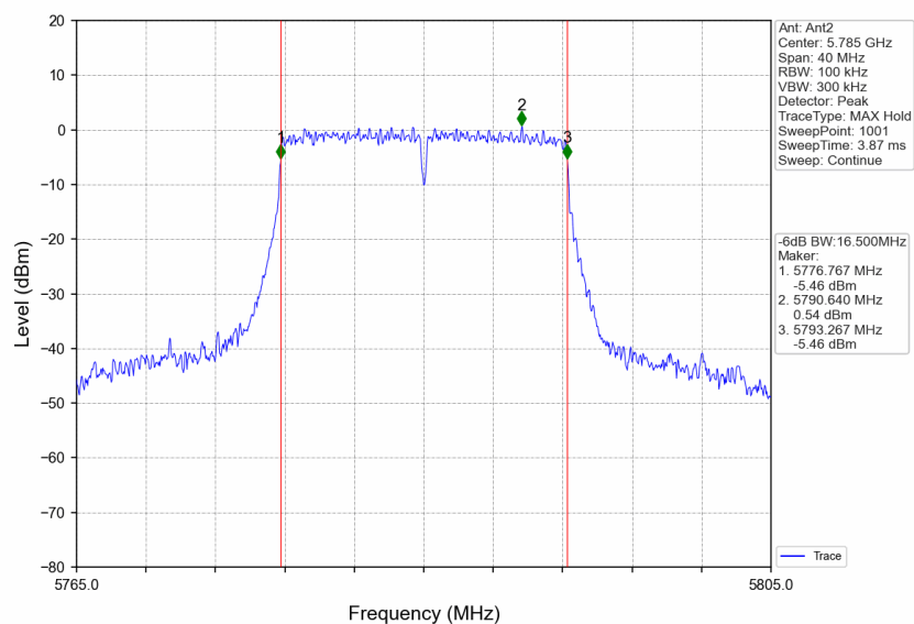
802.11a_MCH_5785MHz_Ant2_NTNV
