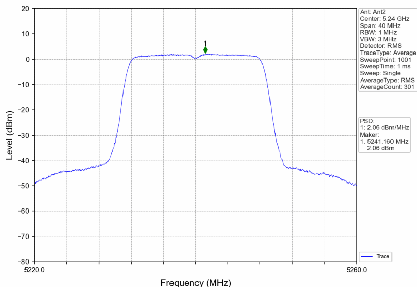
802.11a_HCH_5240MHz_Ant2_NTNV
