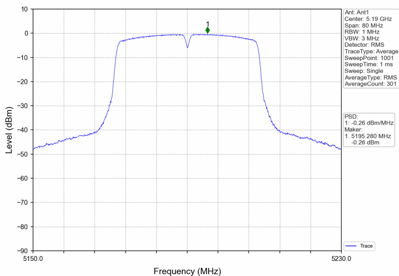
802.11n(HT40)_LCH_5190MHz_Ant1_NTNV
