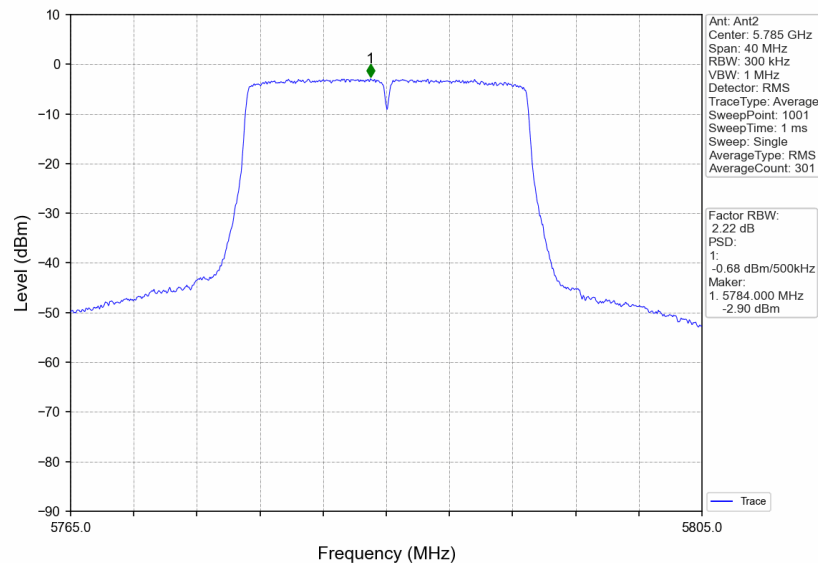
802.11ac(VHT20) MCH_5785MHz_Ant2_NTNV
