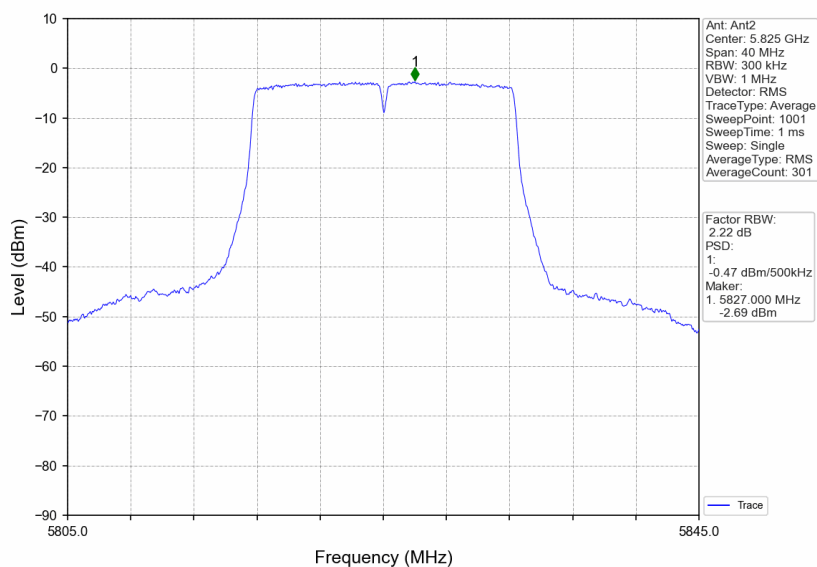
802.11a_HCH_5825MHz_Ant2_NTNV
