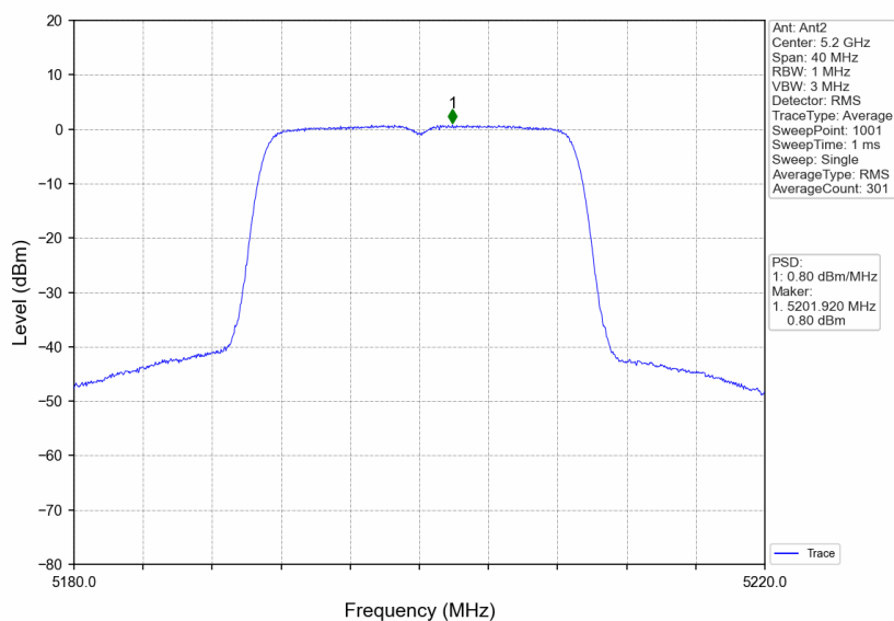
802.11ac(VHT20) MCH 5200MHz Ant2 NTNV
