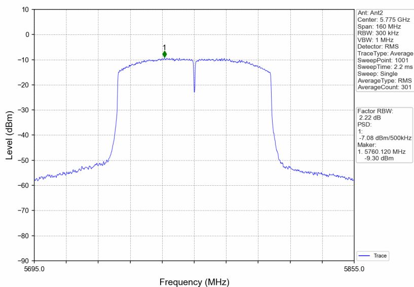
802.11ac(VHT80) MCH_5775MHz_Ant2_NTNV
