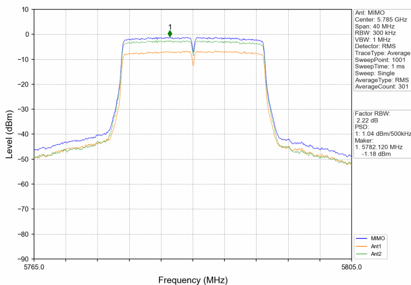
802.11n(HT20)_MCH_5785MHz_MIMO_NTNV
