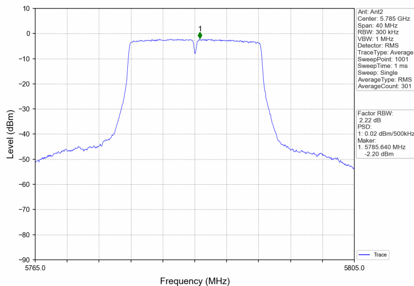
802.11a_MCH_5785MHz_Ant2_NTNV
