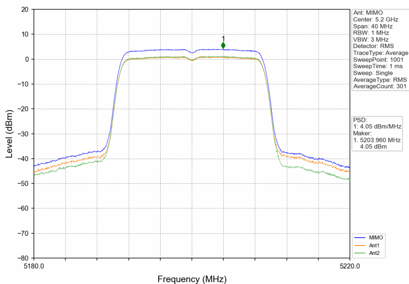
802.11n(HT20)_MCH_5200MHz_MIMO_NTNV
