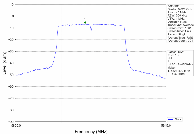
802.11ac(VHT20) HCH_5825MHz_Ant1_NTNV
