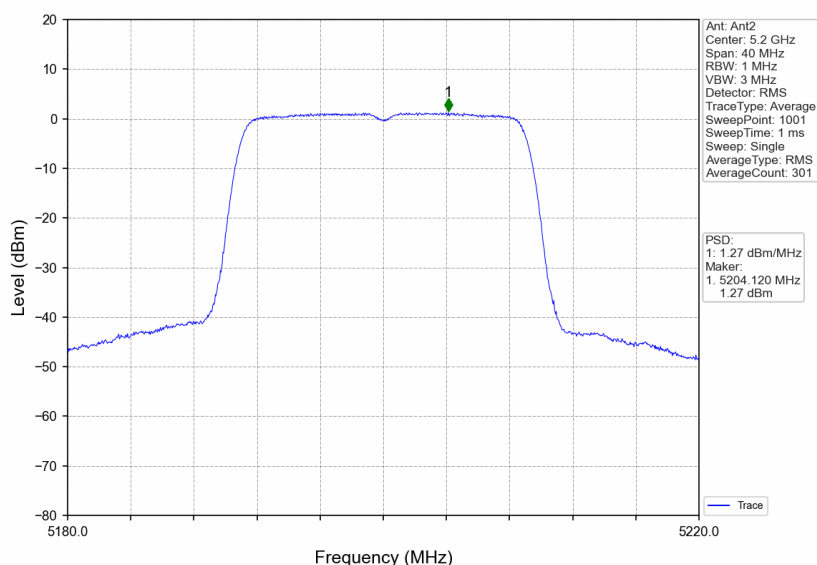
802.11n(HT20)_MCH_5200MHz_MIMO_NTNV
