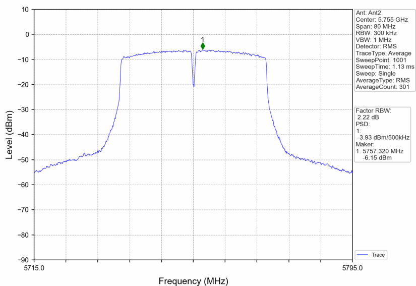
802.11ac(VHT40)_LCH_5755MHz_Ant2_NTNV
