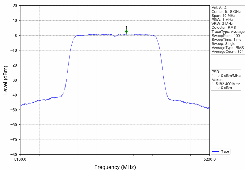
802.11n(HT20)_LCH_5180MHz_Ant2_NTNV
