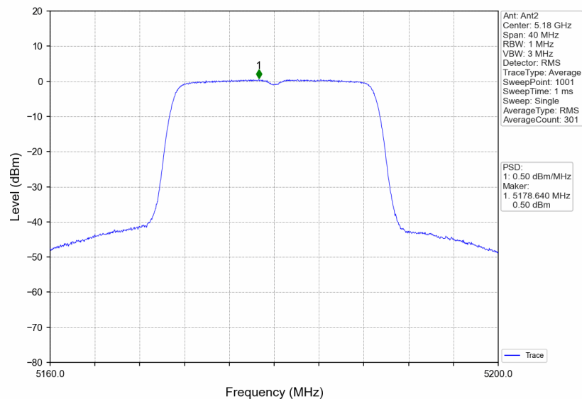
802.11ac(VHT20) LCH 5180MHz MIMO_NTNV
