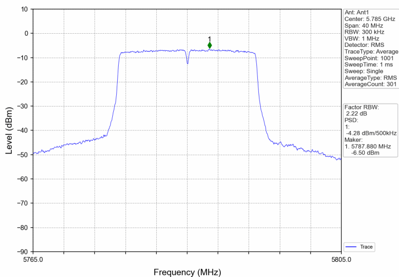
802.11n(HT20)_MCH_5785MHz_Ant1_NTNV
