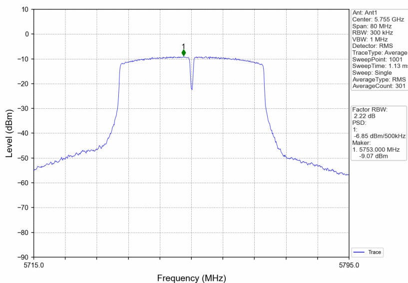
802.11n(HT40)_LCH_5755MHz_Ant1_NTNV
