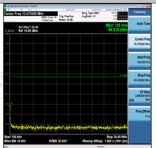
Band2-3MHz-16QAM-18900-1RB#14-0.15~30-P ASS
