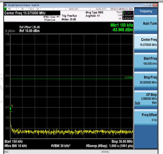
Band2-3MHz-16QAM-18615-1RB#14-0.15~30-P ASS
