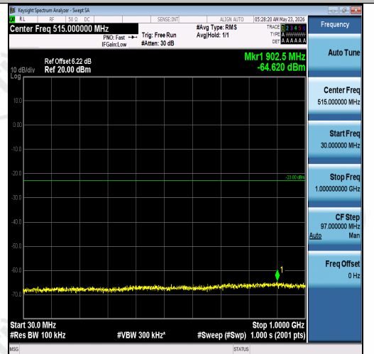
Band2-3MHz-QPSK-18900-1RB#14-30~1000-P ASS
