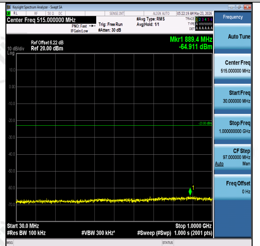
Band2-3MHz-QPSK-18615-1RB#14-30~1000-P-ASS
