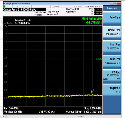
Band2-3MHz-QPSK-19185-1RB#14-30~1000-P ASS
