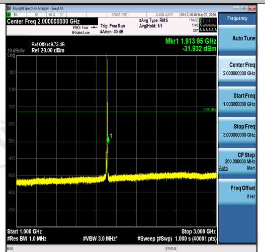
Band2-5MHz-QPSK-19175-1RB#0-1000~3000-P ASS
