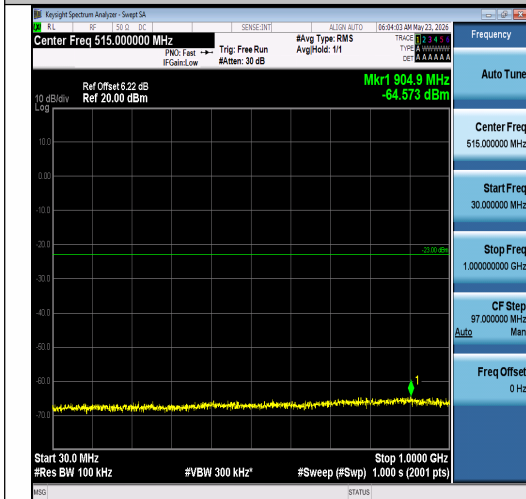
Band2-5MHz-QPSK-18625-25RB#0-30~1000-P ASS
