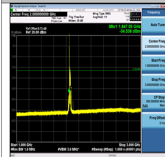
Band2-20MHz-16QAM-18700-1RB#0-1000~300 0-PASS
