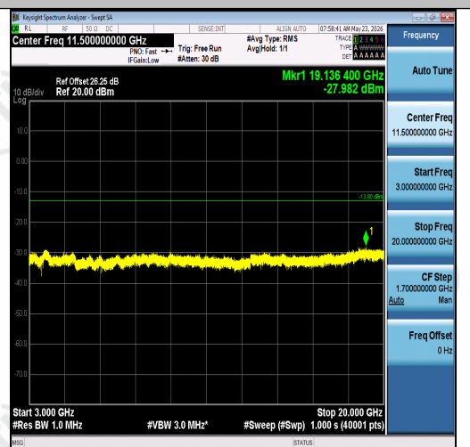
Band2-20MHz-16QAM-18700-1RB#0-3000~200 00-PASS
