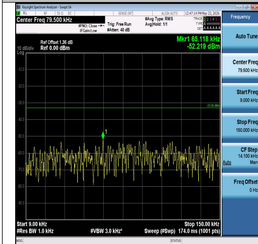
Band26(824-849)-5MHz-QPSK-27015-1RB#0-0. 009~0.15-PASS
