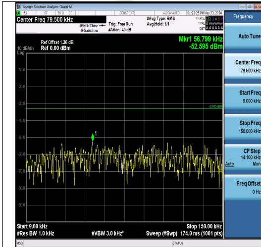
Band26(824-849)-10MHz-QPSK-26915-50RB#0-0.009~0.15-PASS
