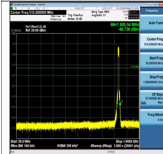
Band26(824-849)-10MHz-QPSK-26915-50RB#0-30~1000-PASS
