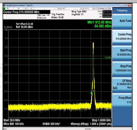
Band26(824-849)-10MHz-16QAM-26840-50RB# 0-30~1000-PASS
