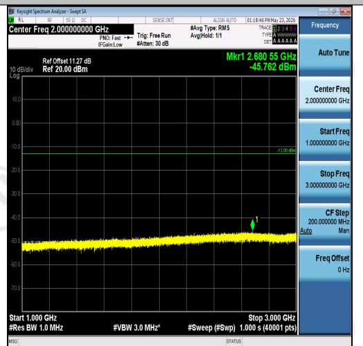
Band26(824-849)-10MHz-QPSK-26915-1RB#0-1 000~3000-PASS
