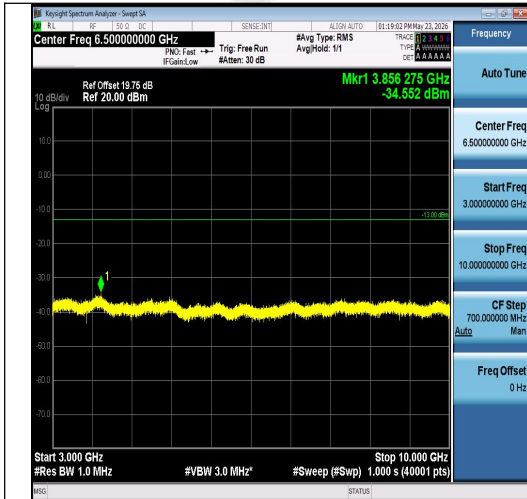
Band26(824-849)-10MHz-QPSK-26915-1RB#0-3 000~10000-PASS
