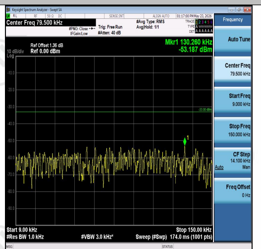
Band26(824-849)-10MHz-16QAM-26840-50RB# 0-0.009~0.15-PASS
