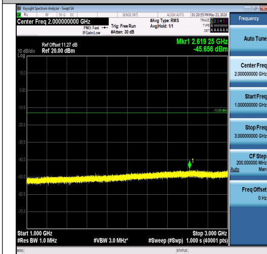
Band26(824-849)-10MHz-QPSK-26915-1RB#49- 1000~3000-PASS
