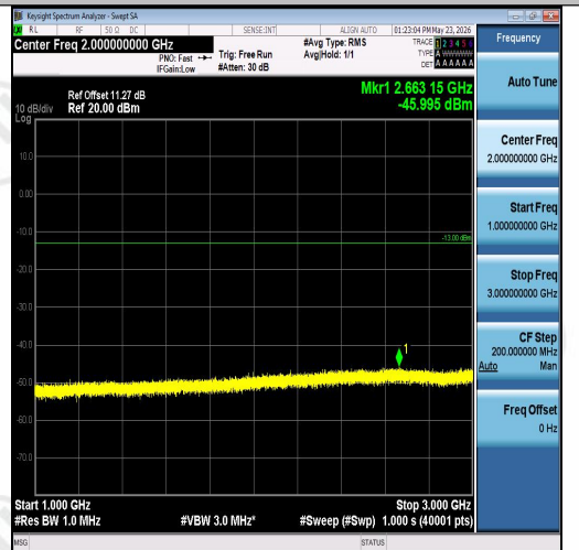
Band26(824-849)-10MHz-QPSK-26915-50RB#0-1000~3000-PASS
