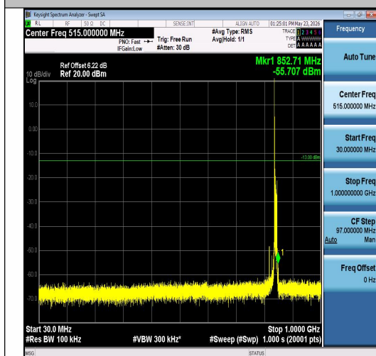
Band26(824-849)-10MHz-QPSK-26990-1RB#0-3 0~1000-PASS
