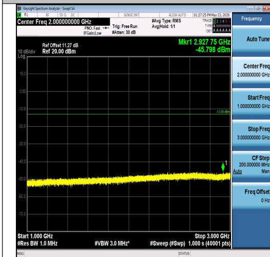
Band26(824-849)-10MHz-QPSK-26990-1RB#49- 1000~3000-PASS
