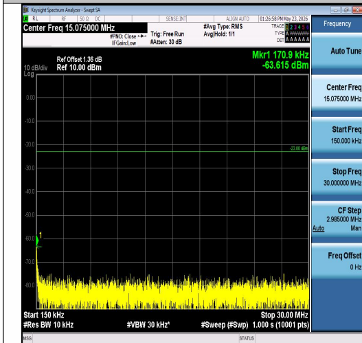
Band26(824-849)-10MHz-QPSK-26990-1RB#49- 0.15~30-PASS
