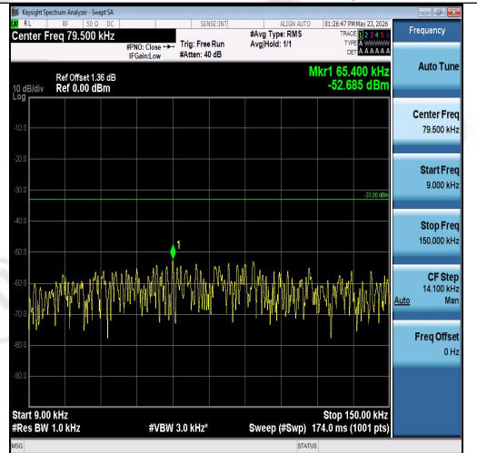
Band26(824-849)-10MHz-QPSK-26990-1RB#49- 0.009~0.15-PASS
