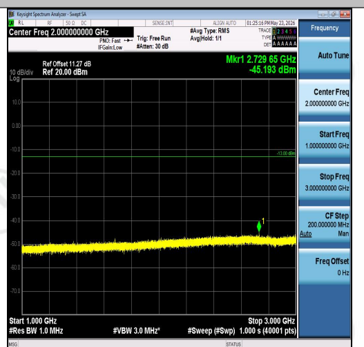
Band26(824-849)-10MHz-QPSK-26990-1RB#0-1 000~3000-PASS
