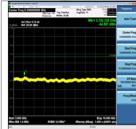
Band26(824-849)-10MHz-QPSK-26990-1RB#0-3 000~10000-PASS
