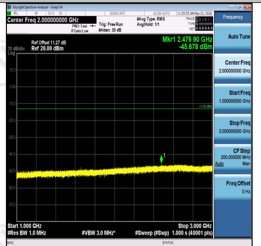
Band26(824-849)-1.4MHz-QPSK-26797-1RB#0-1000~3000-PASS
