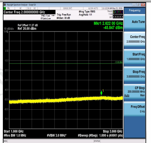
Band26(824-849)-1.4MHz-QPSK-26915-1RB#0- 1000~3000-PASS
