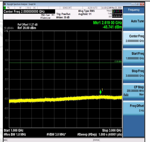
Band26(824-849)-1.4MHz-QPSK-26797-6RB#0-1000~3000-PASS
