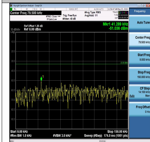
Band26(824-849)-3MHz-QPSK-26805-1RB#0-0. 009~0.15-PASS
