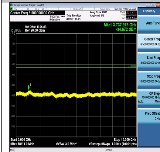
Band26(824-849)-3MHz-QPSK-26805-15RB#0-3 000~10000-PASS
