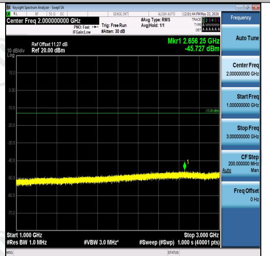
Band26(824-849)-3MHz-QPSK-26805-15RB#0-1 000~3000-PASS
