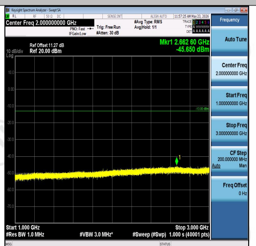
Band26(824-849)-3MHz-QPSK-26805-1RB#0-10 00~3000-PASS
