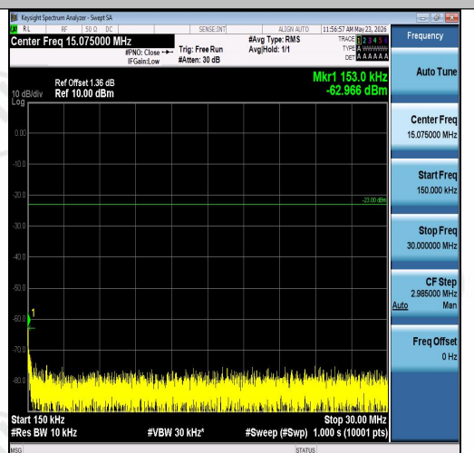
Band26(824-849)-3MHz-QPSK-26805-1RB#0-0. 15~30-PASS
