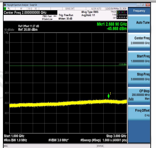
Band26(824-849)-3MHz-QPSK-26915-1RB#0-10 00~3000-PASS
