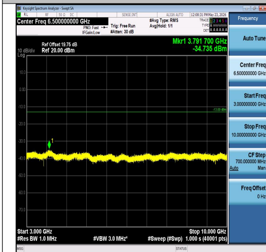
Band26(824-849)-3MHz-QPSK-26915-15RB#0-3 000~10000-PASS
