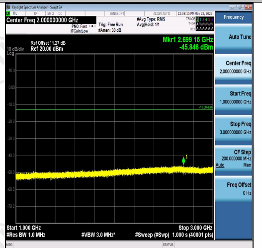
Band26(824-849)-3MHz-QPSK-26915-15RB#0-1 000~3000-PASS
