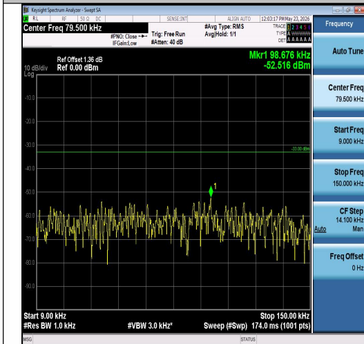
Band26(824-849)-3MHz-QPSK-26915-1RB#0-0. 009~0.15-PASS
