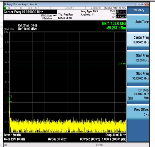
Band26(824-849)-3MHz-QPSK-26915-1RB#0-0. 15~30-PASS
