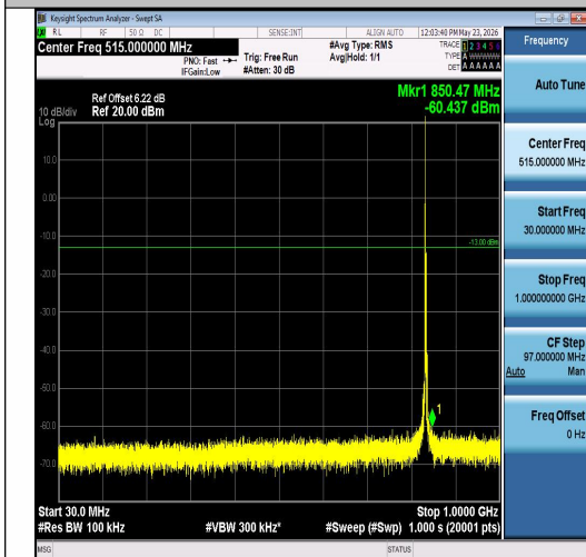
Band26(824-849)-3MHz-QPSK-26915-1RB#0-30 ~1000-PASS
