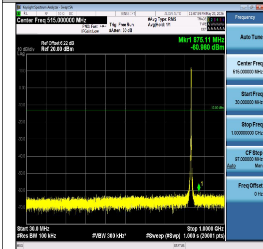
Band26(824-849)-3MHz-QPSK-26915-15RB#0-3 0~1000-PASS
