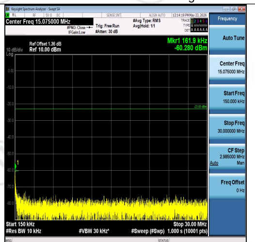
Band26(824-849)-3MHz-QPSK-27025-15RB#0-0 .15~30-PASS
