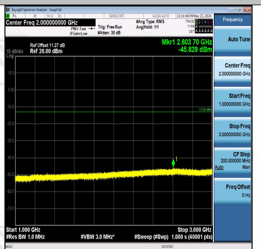
Band26(824-849)-3MHz-QPSK-27025-15RB#0-1 000~3000-PASS
