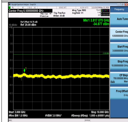
Band26(824-849)-3MHz-QPSK-27025-15RB#0-3 000~10000-PASS
