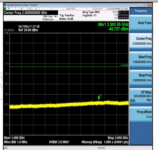
Band26(824-849)-3MHz-QPSK-27025-1RB#0-10 00~3000-PASS
