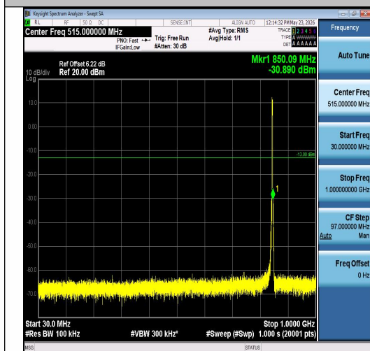
Band26(824-849)-3MHz-QPSK-27025-15RB#0-3 0~1000-PASS
