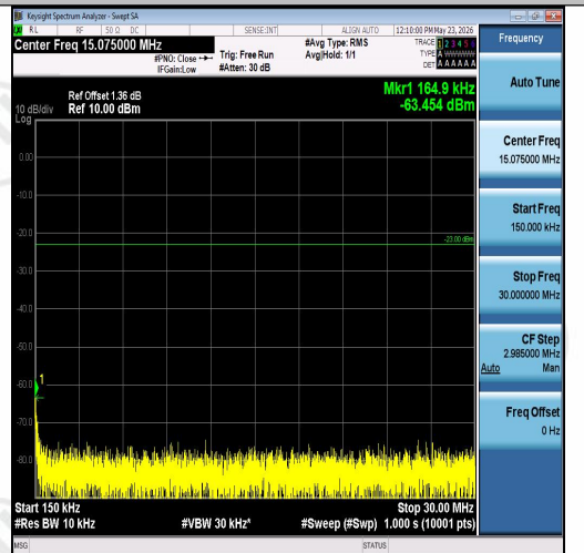
Band26(824-849)-3MHz-QPSK-27025-1RB#0-0. 15~30-PASS
