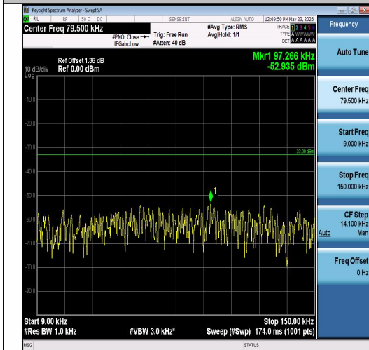
Band26(824-849)-3MHz-QPSK-27025-1RB#0-0. 009~0.15-PASS
