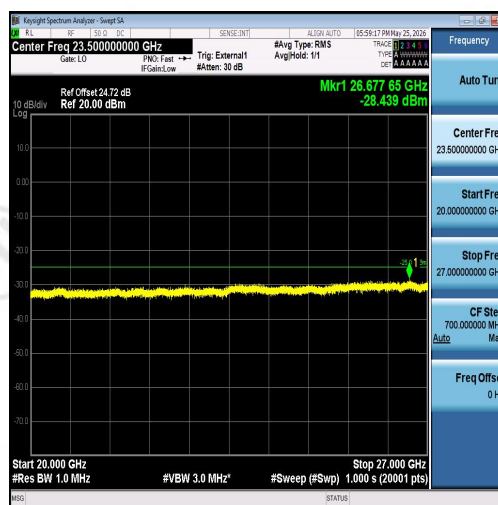
Band41-10MHz-QPSK-39700-50RB#0-20000~27000-PASS
