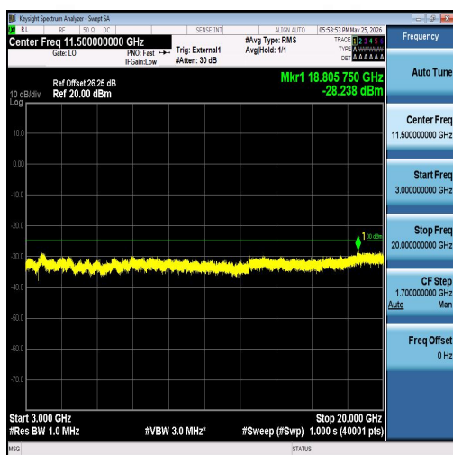
Band41-10MHz-QPSK-39700-50RB#0-3000~20000-PASS
