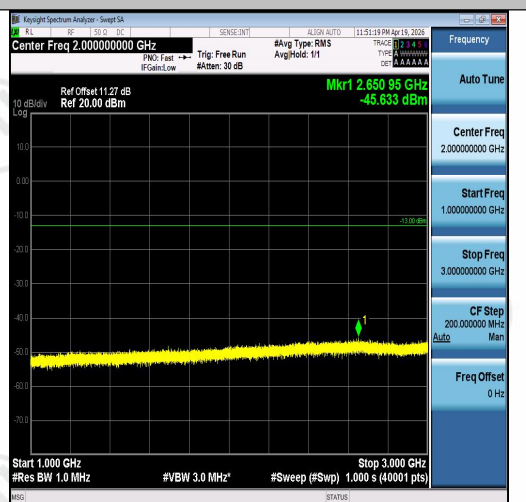
Band5-3MHz-QPSK-20635-1RB#0-1000~3000-P ASS
