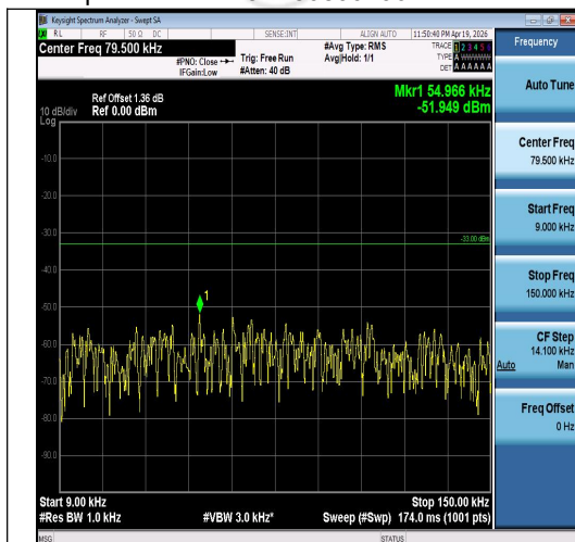
Band5-3MHz-QPSK-20635-1RB#0-0.009~0.15-P ASS
