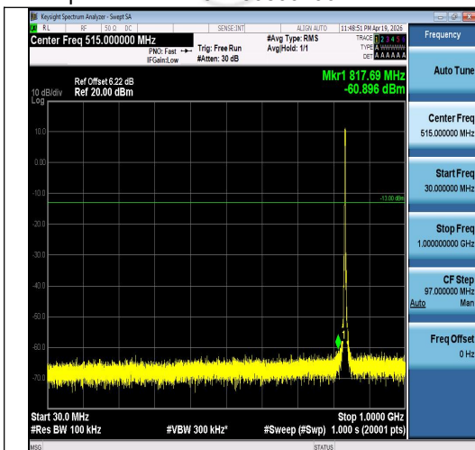
Band5-3MHz-QPSK-20525-15RB#0-30~1000-P ASS
