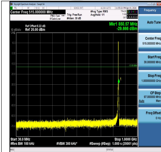
Band5-3MHz-QPSK-20635-15RB#0-30~1000-P ASS
