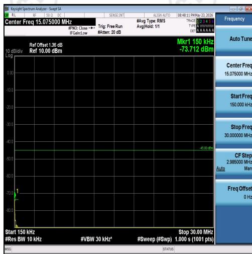
Band7-15MHz-16QAM-20825-1RB#0-20000~27 000-PASS
