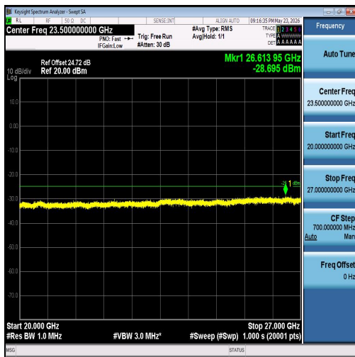
Band7-20MHz-QPSK-20850-100RB#0-20000~2 7000-PASS
