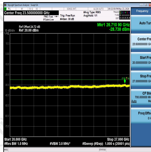
Band7-20MHz-QPSK-21350-100RB#0-20000~27000-PASS
