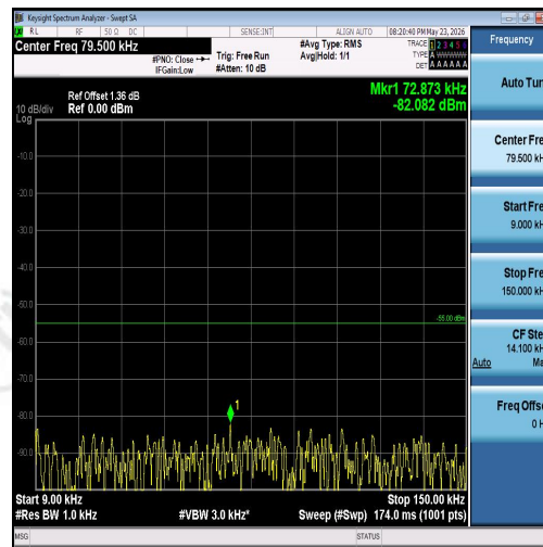
Band7-10MHz-QPSK-20800-50RB#0-0.009~0.15-PASS
