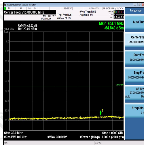
Band7-10MHz-QPSK-20800-50RB#0-30~1000-PASS
