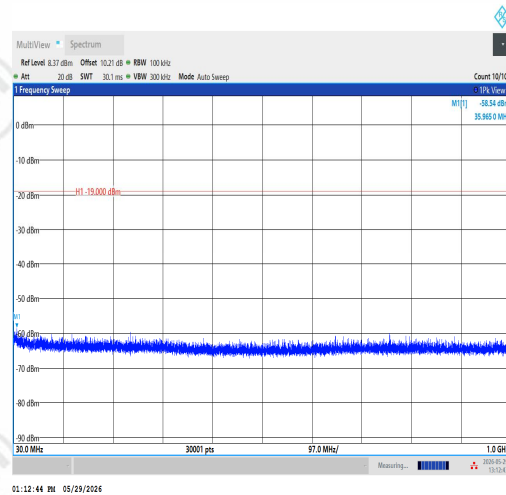
11G-Ant1-2462-30~1000-PASS
