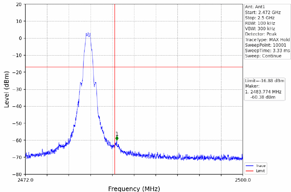
1M_HCH_2480MHz_DataRate=_Ant1_NTNV
